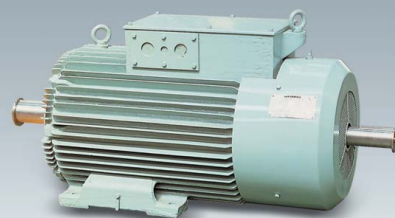
권선형 전폐 크레인 전동기
